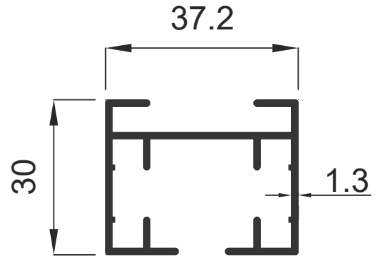
1264 0.561 Kg / m
