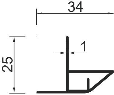
2585 0.242 Kg / m
