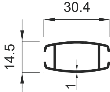
1537 0.241 Kg / m
