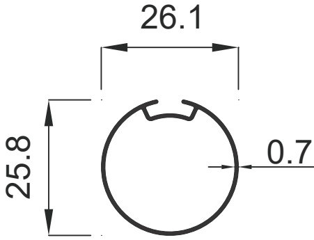
2216 0.168 Kg / m
