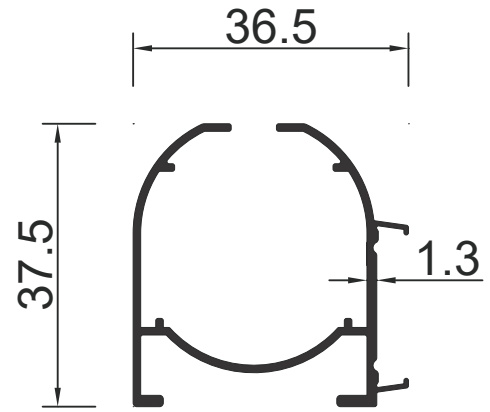
2099 0.407 Kg / m
