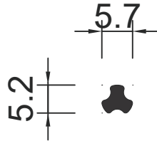
1746 0.050 Kg / m
