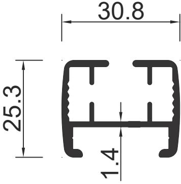
2222 0.515 Kg / m
