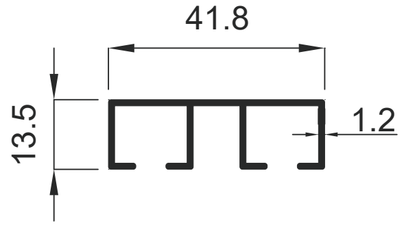
2088 0.347 Kg / m
