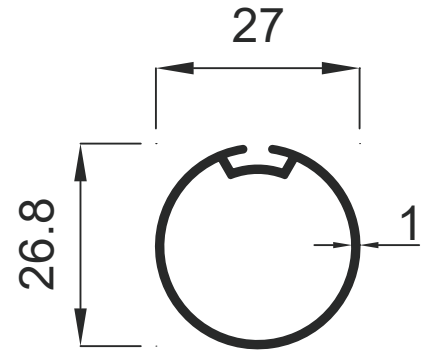
232 0.243 Kg / m
