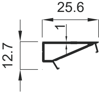
1950 0.170 Kg / m
